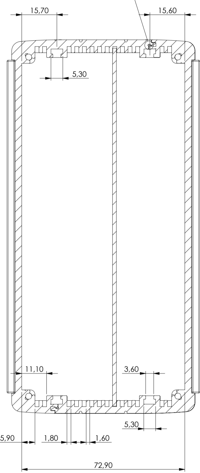
SEZIONE B-B
